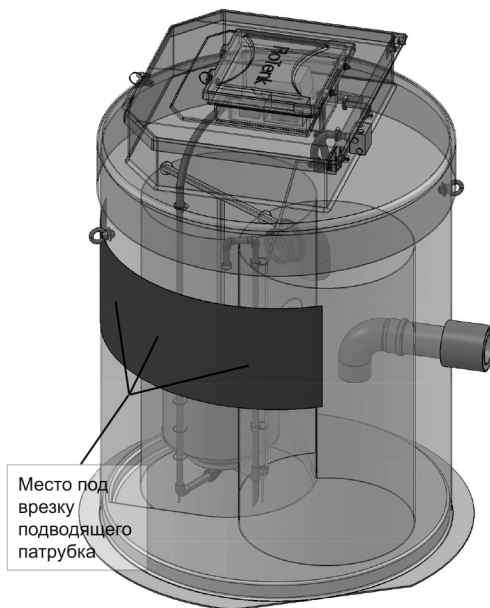
Рис. 1 Схема станции FloTenk-BioPurit
