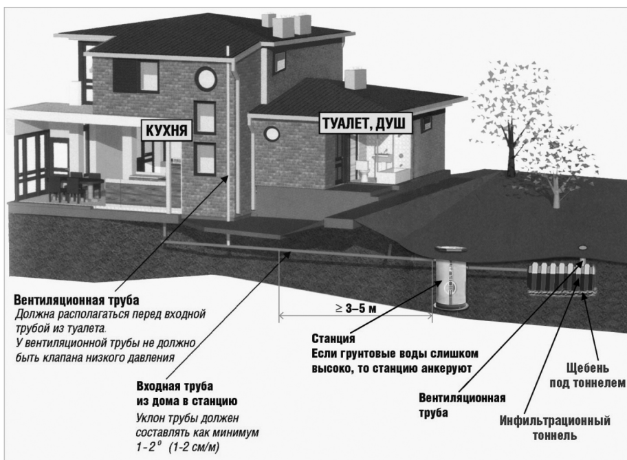
Рис. 2 Схема установки станции FloTenk-BioPurit
