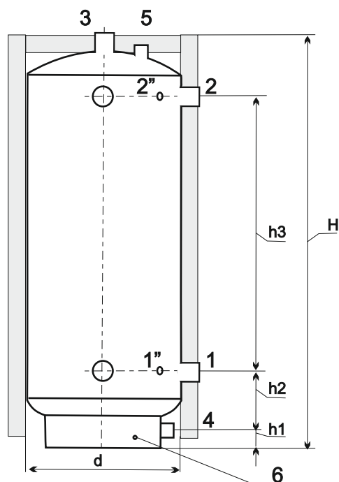
Рисунок 1. Схема подключения теплоаккумулятора серии TA 200
