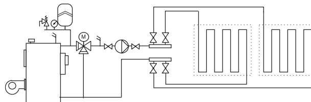
Рис. 25 Система «теплых полов»
