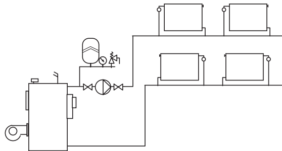
Рис. 23 Однотрубная система отопления
