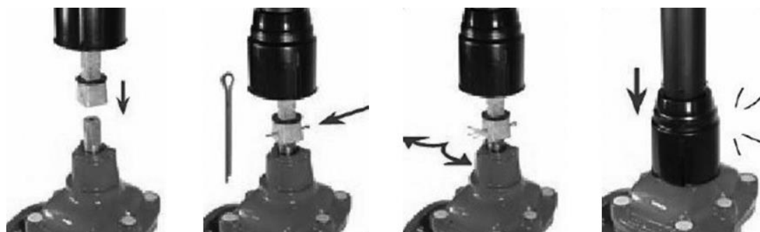
Рис. 4 Порядок установки телескопического штока на задвижку.
