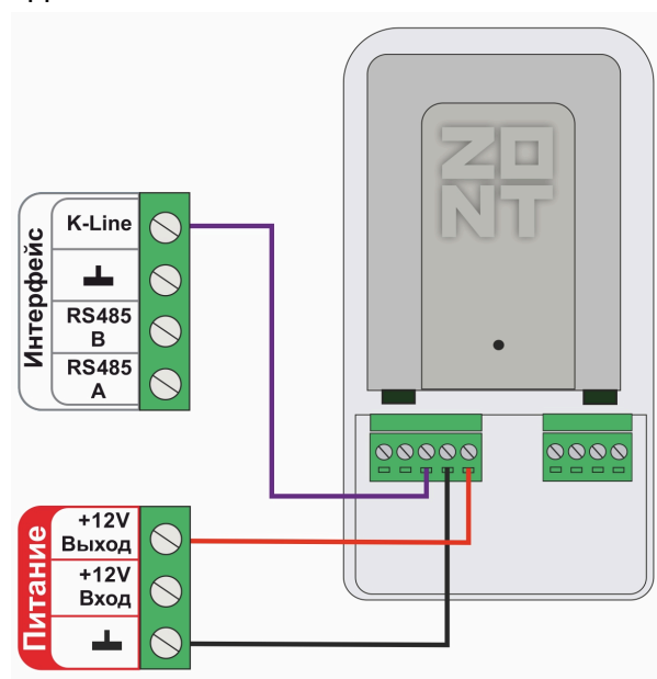
Схема подключения внешнего адаптера цифровой шины ECO по K-Line :
